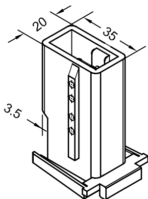
Art. 248646 blanco RAU-PA + 30% fibra de vidrio Unión mecánica con junta para poste 78 (E 1:2)
