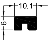
Art. 261699 blanco, marrón Pieza de fijación para unión mecánica universal
